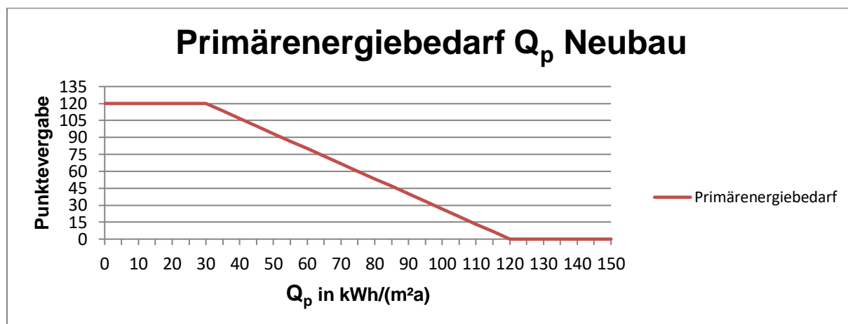
Grafik 7: Punktvergabe in Abhängigkeit vom Primärenergiebedarf
