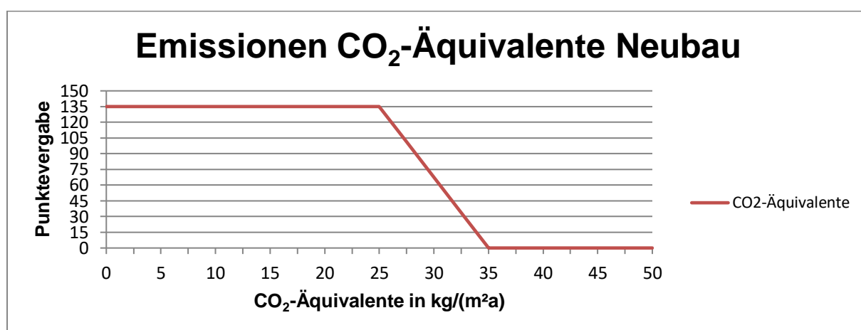
Grafik 8: Punktvergabe in Abhängigkeit der Emissionen in CO 2 -Äquivalente
