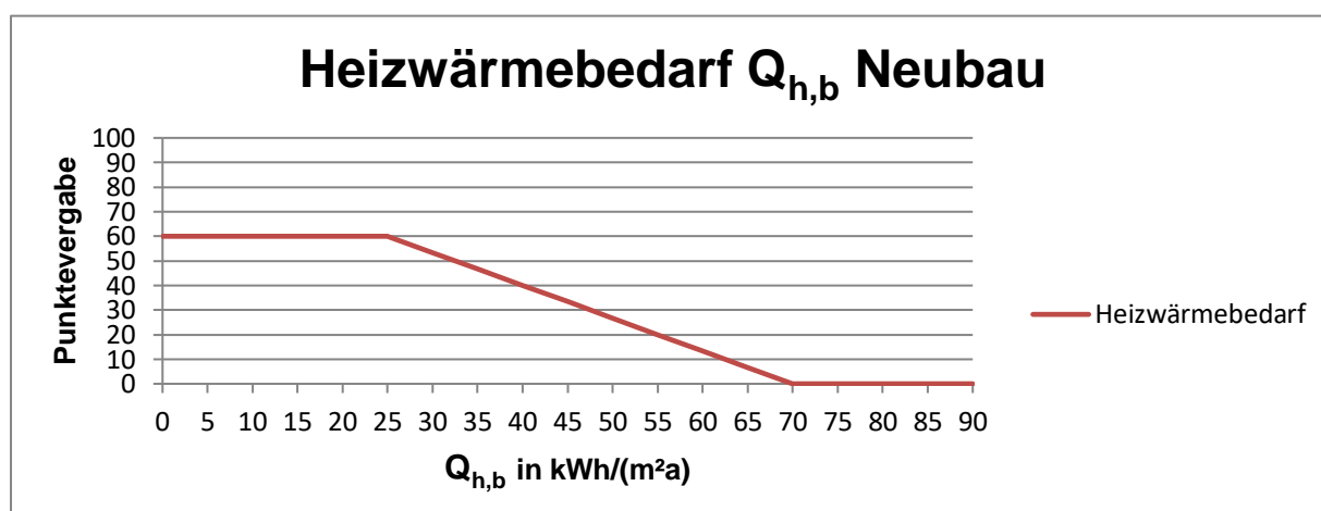
Grafik 5: Punktvergabe in Abhängigkeit vom Heizwärmebedarf
