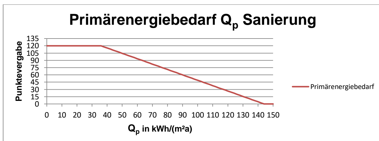
Grafik 16: Punktvergabe in Abhängigkeit vom Primärenergiebedarf
