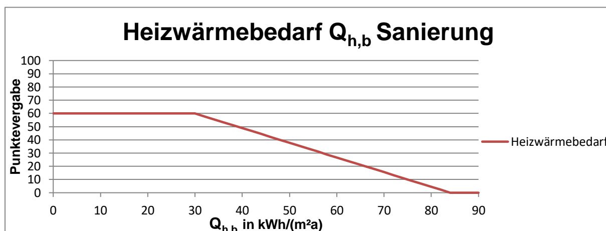
Grafik 14: Punktvergabe in Abhängigkeit vom Heizwärmebedarf
