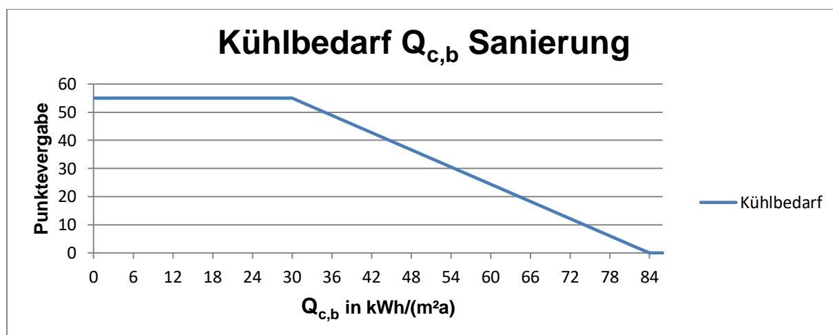
Grafik 15: Punktevergabe in Abhängigkeit vom Kühlbedarf
