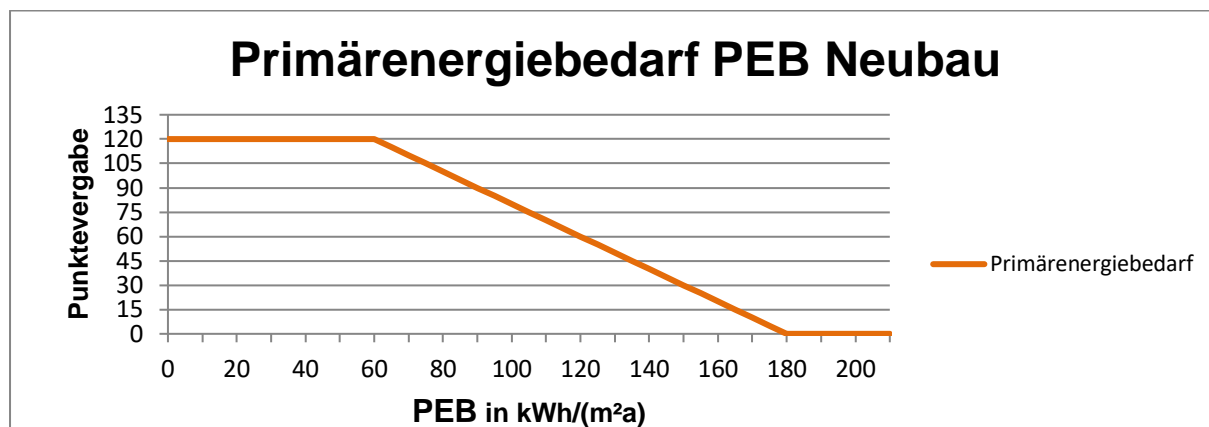
Grafik 2: Punktevergabe in Abhängigkeit vom Primärenergiekennwert PHPP
